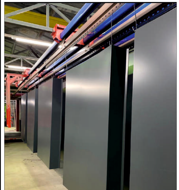
Покраска крупногабаритных доборных элементов кровли
